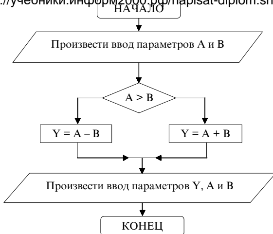
Рис. 8.2.2. Алгоритм вычисления функции
