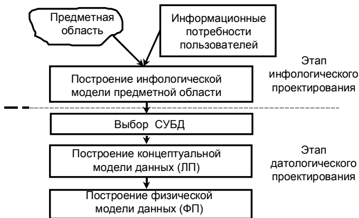
Рис. 9.1.3. Этапы проектирования БД
