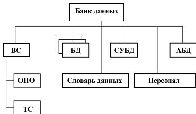
Рис. 9.1.1. Основные компоненты БД
