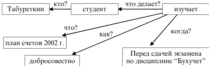
Рис. 10.2.7. Семантическая сеть для предложения (ситуации)
