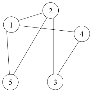
Рис. 1.3.1. Неориентированный граф
