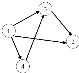
Рис. 1.3.2. Ориентированный граф
