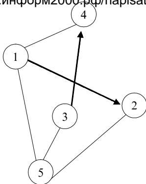
Рис. 1.3.3. Смешанный граф
