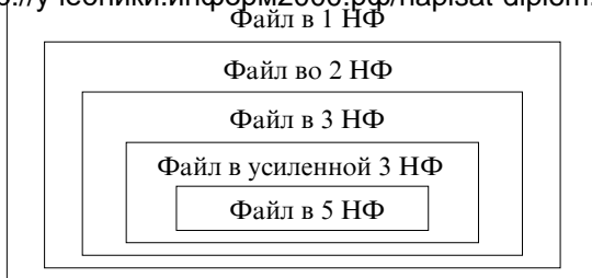
Рис. 9.2.1. Соотношение нормальных форм файлов
